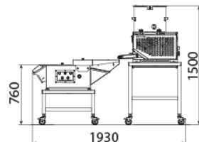
BB 150 + C/E H MAX
